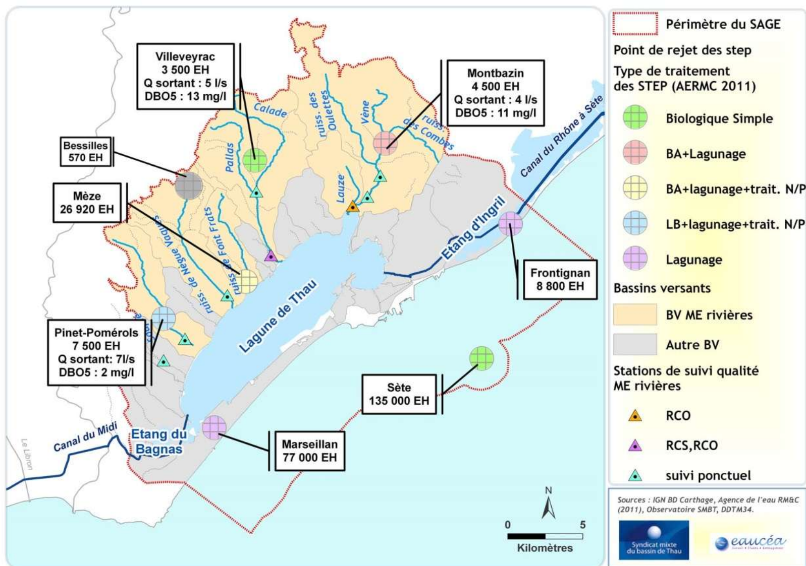
Carte 28 : Caractéristiques des stations d'épuration en 2013 (DDTM 34)
