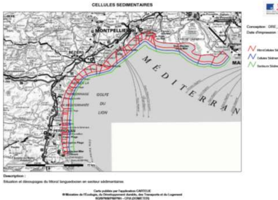
Illustration 20 : les cellules sédimentaires
