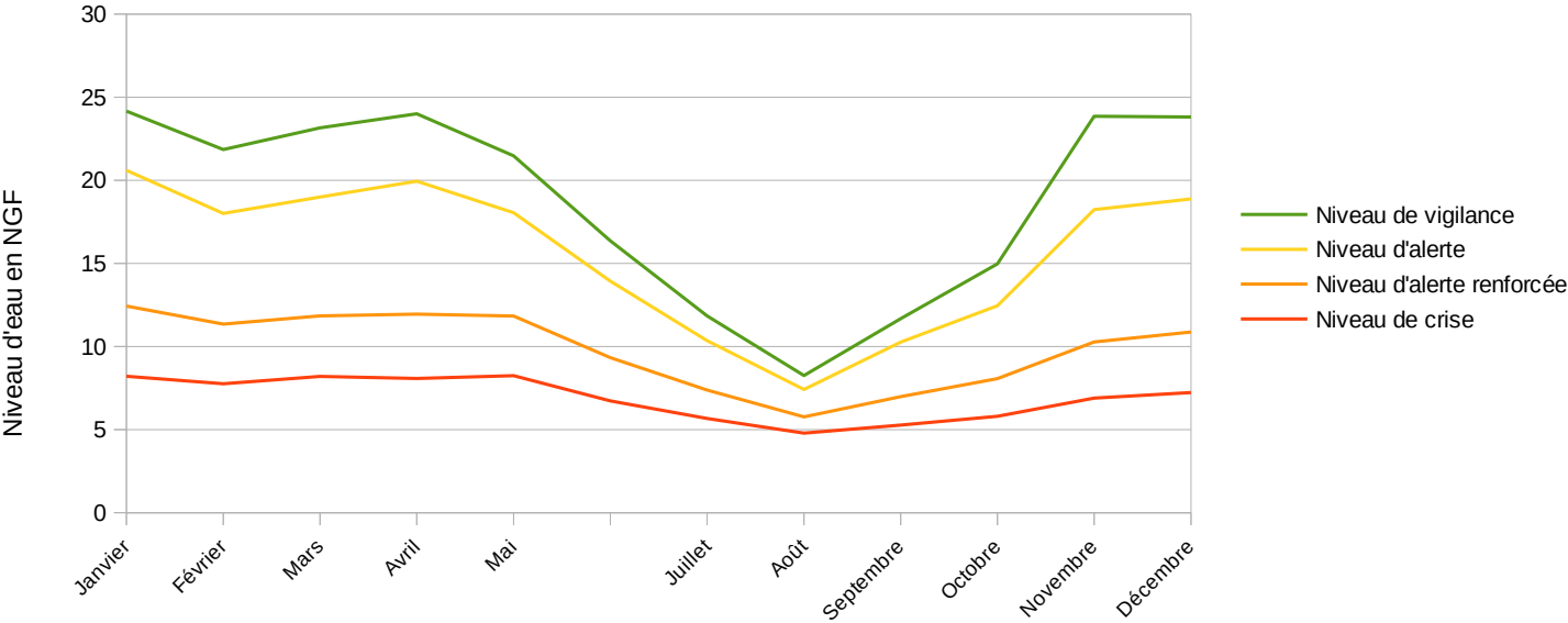
Piézomètre - La Vène à Cournonsec - BSS002JDBC
